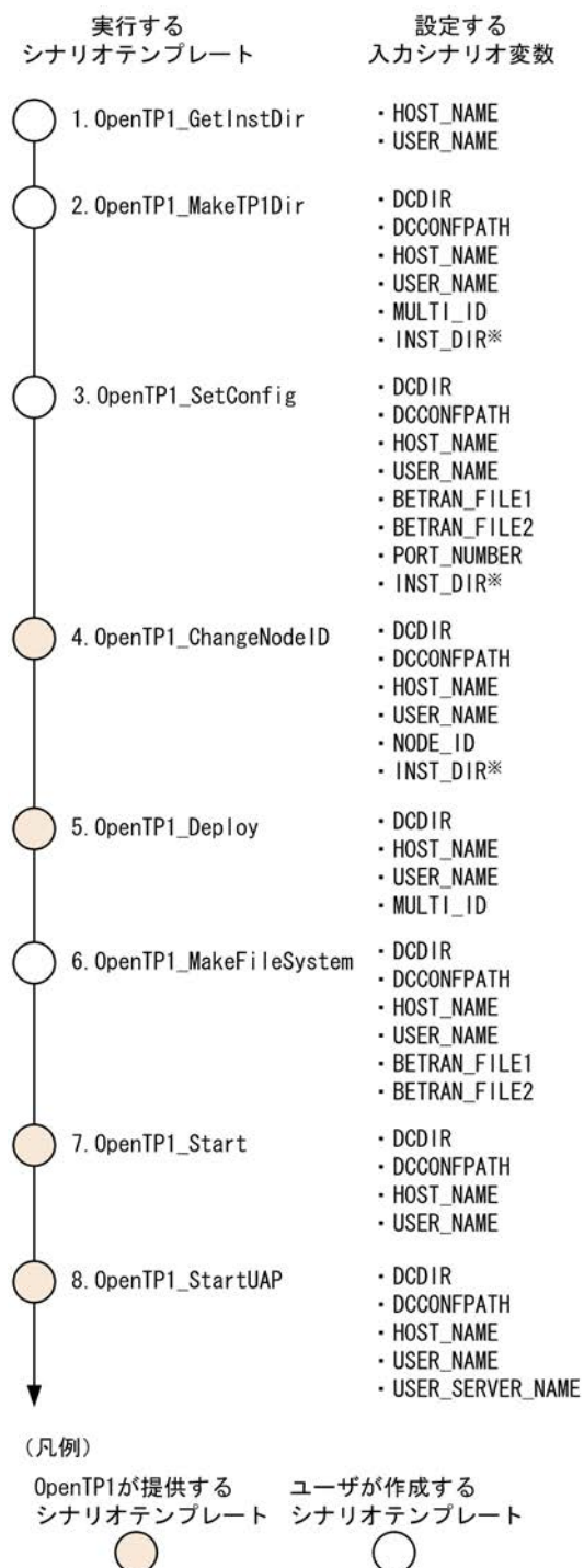
図 6-1 新しい OpenTP1 ノードを追加するシナリオの実行順序
